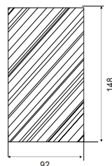
ВЫРЕЗАЕМОЕ ОТВЕРСТИЕ В ДВЕРИ РЕЛЕЙНОГО ШКАФА
