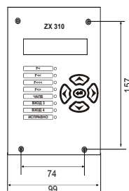
ВИД СПЕРЕДИ
